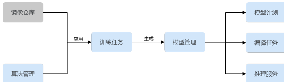
图 6-1 训练服务的开发流程
