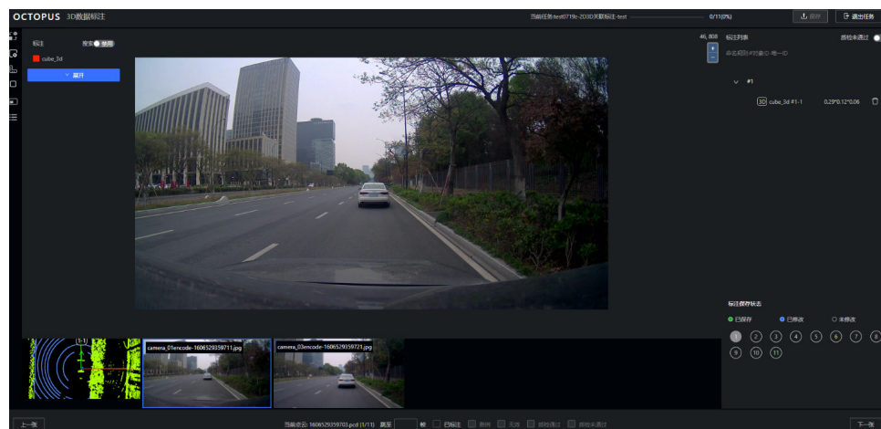
图 5-105 2D3D 关联标注任务
