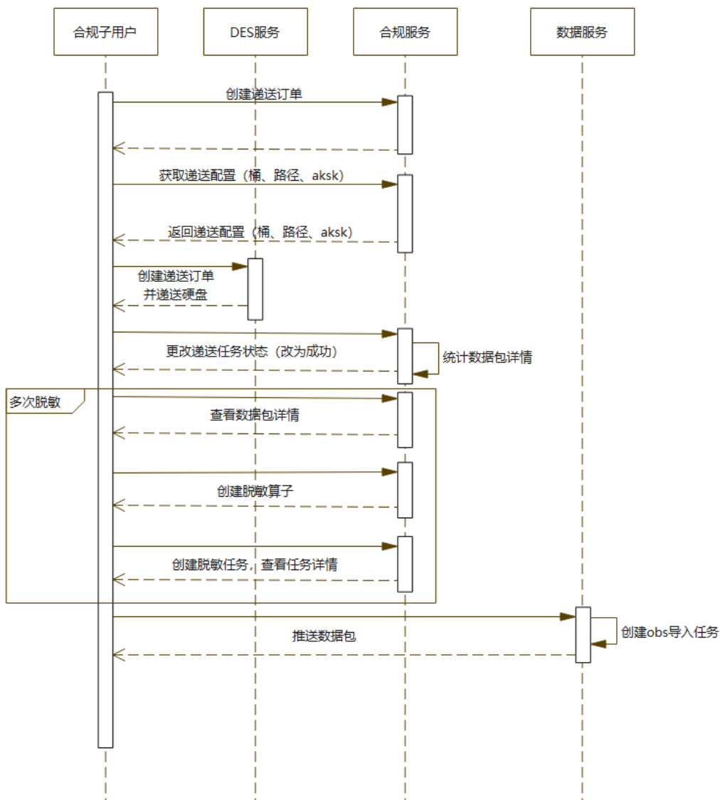
图 3-1 使用合规服务和数据服务时序图
